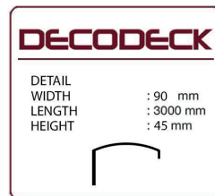
DOOR FRAME
